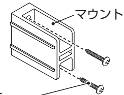
壁取付ねじ左右各2本 (トラスタッピンねじ4×35)
