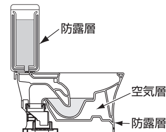
<参考>防露便器、タンクの構造
